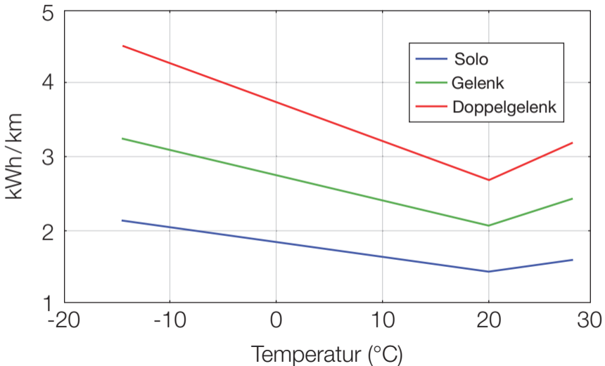
Temperatur-Verbrauchs-Kurve
